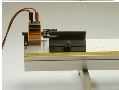
Lanceur pour Banc à Coussin d'Air - ME 912
